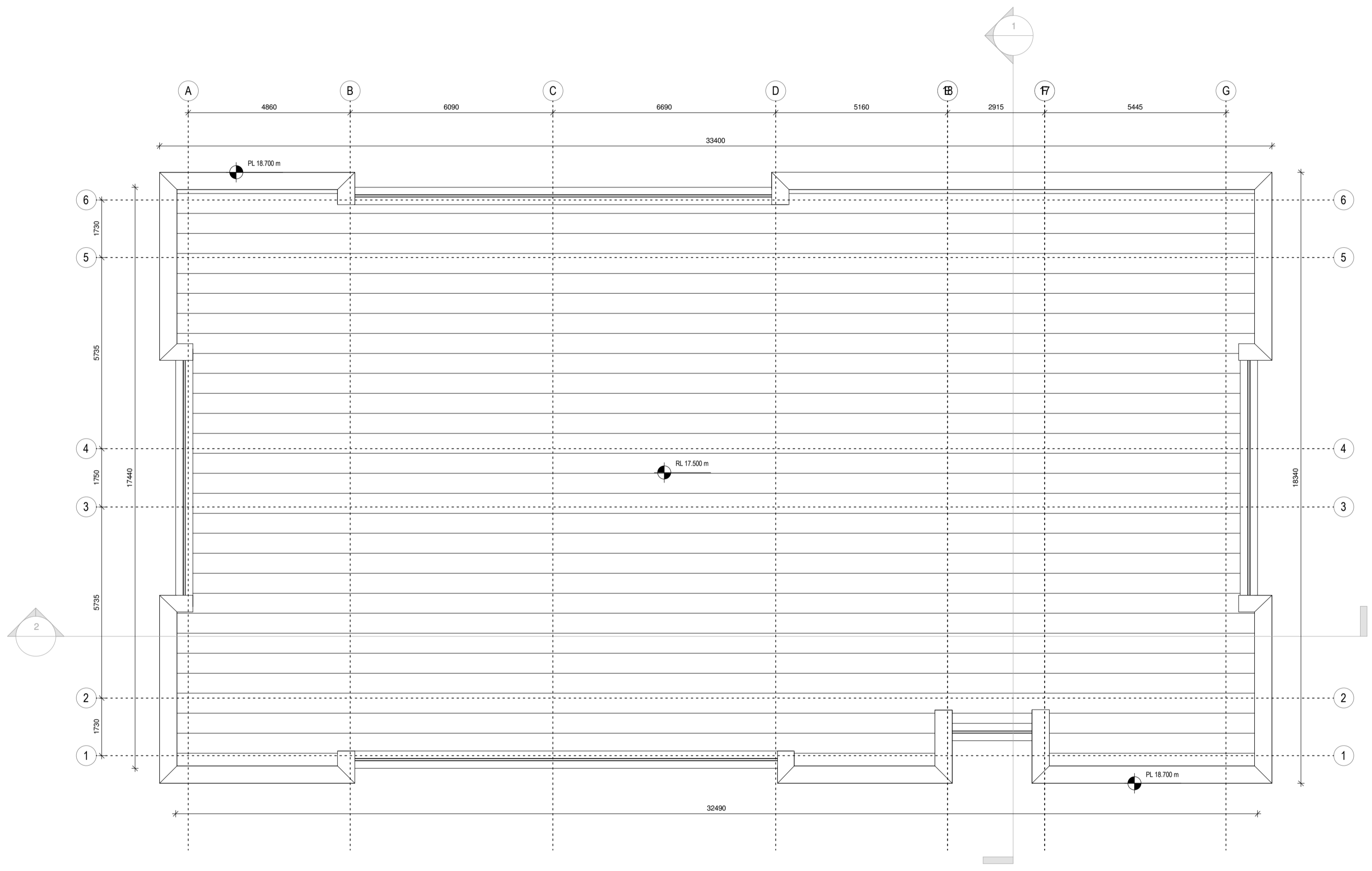
1 L04-01 ROOF LEVEL 1 : 100 1:200@A3
